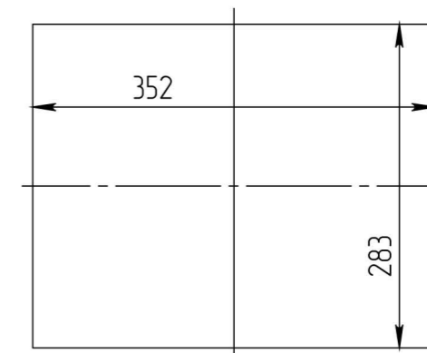
РАЗМЕР ВЫРЕЗА
