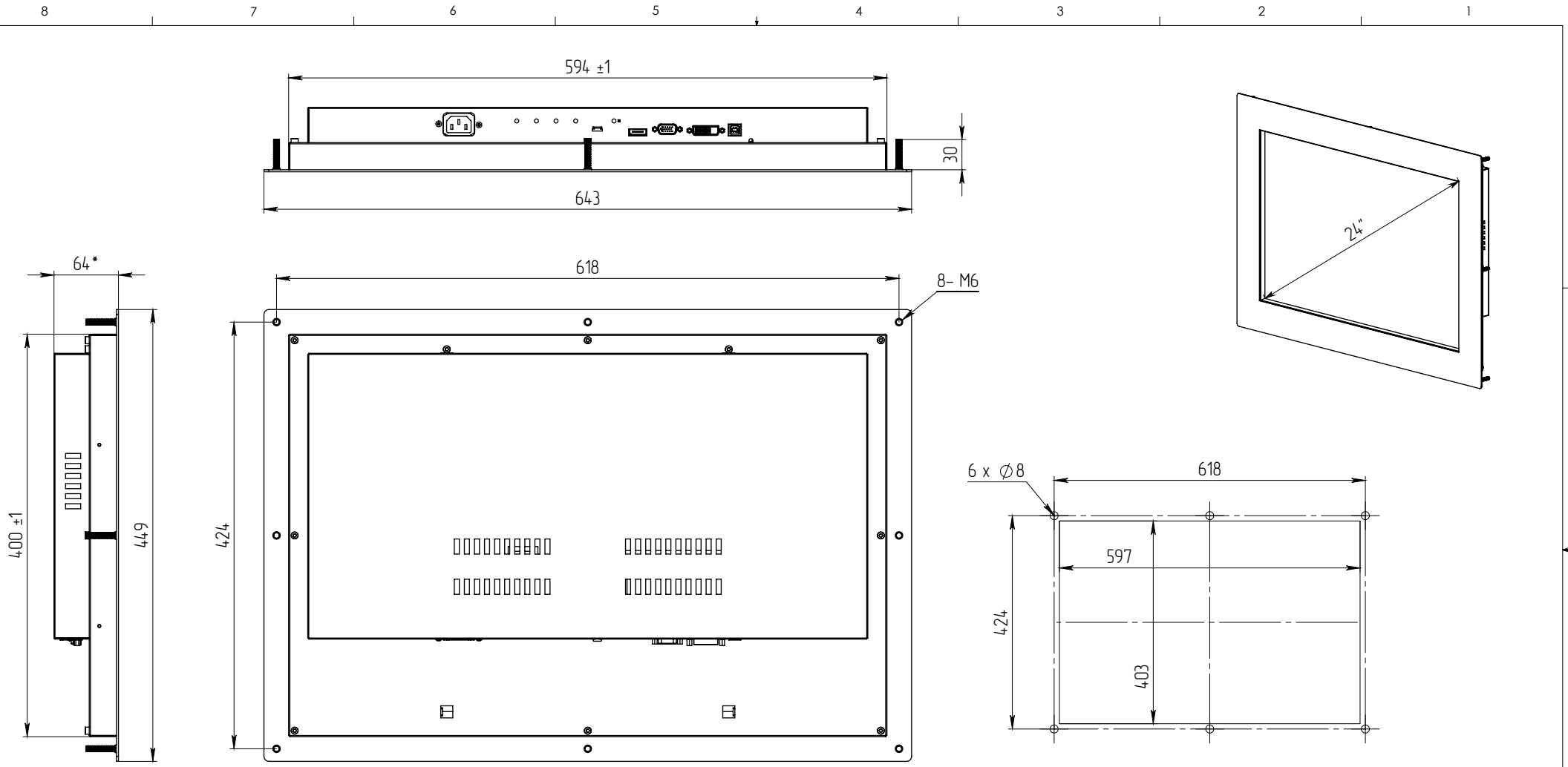
РАЗМЕР ВЫРЕЗА
