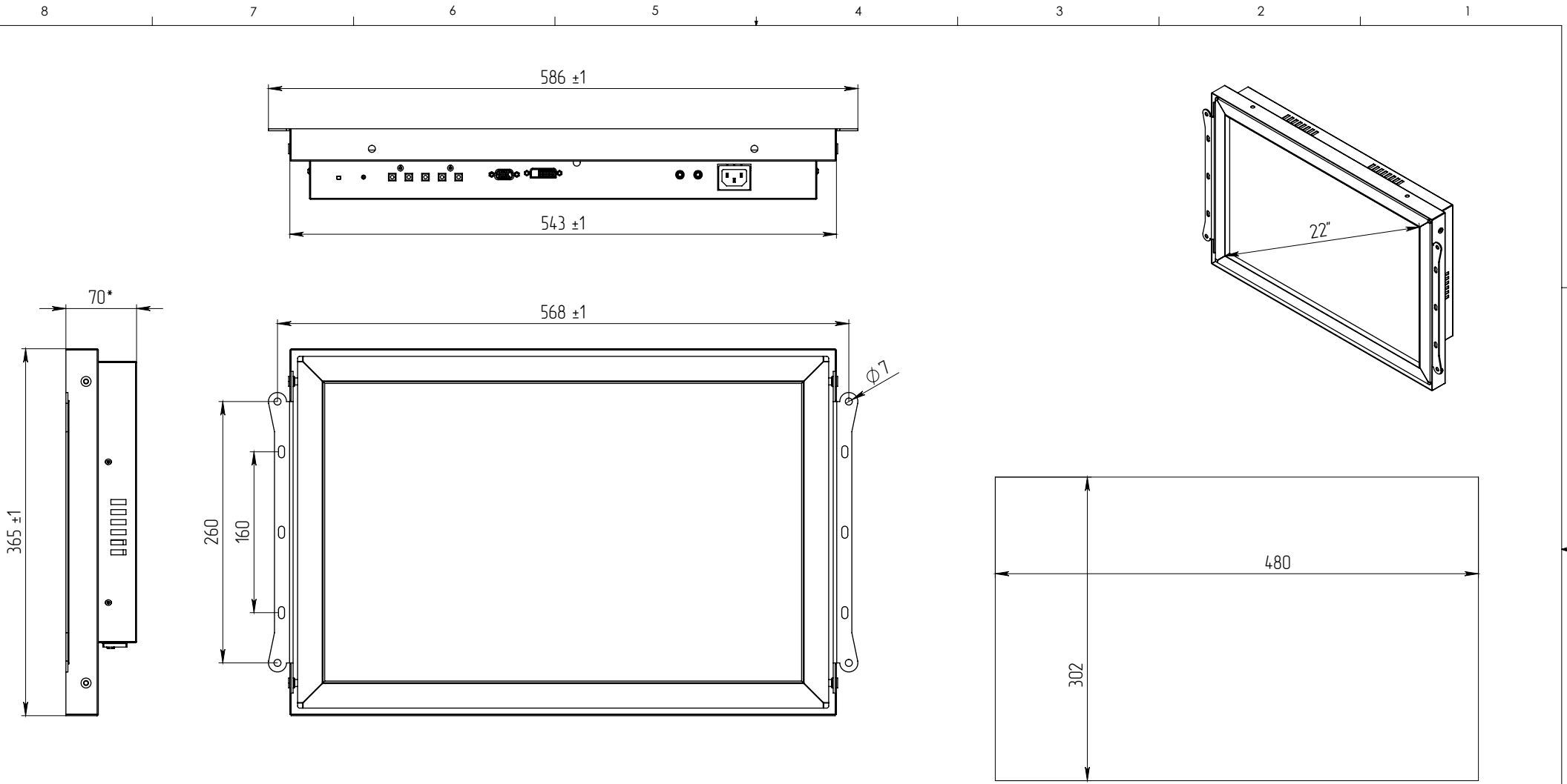
РАЗМЕР ВЫРЕЗА
